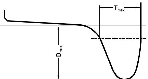
Abb. 3: Maximaler Spurkranz
